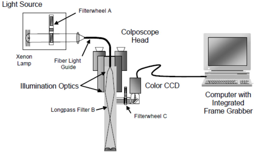
Resim 2. Multispektral Kolposkopi Cihazı
